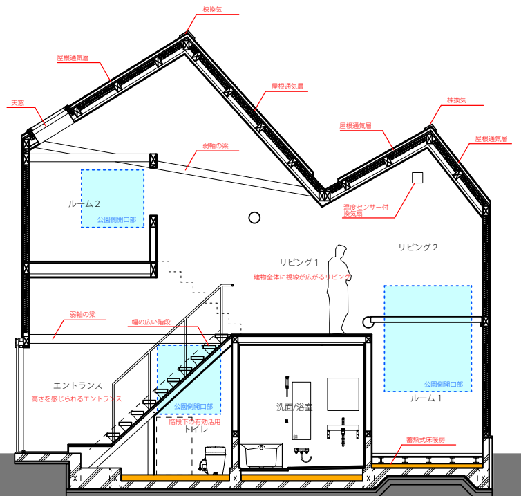
断面図(1/100)
