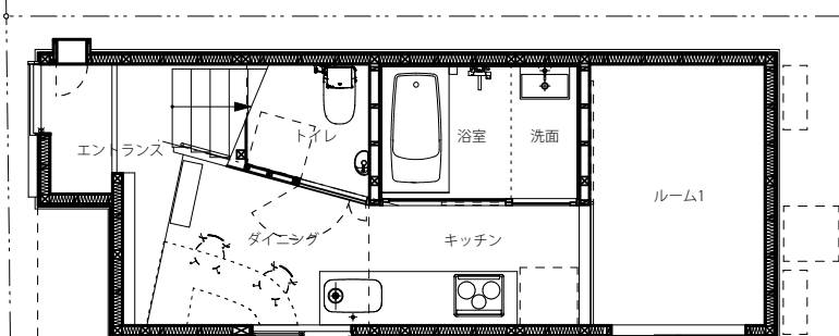
1階平面図(1/100)
