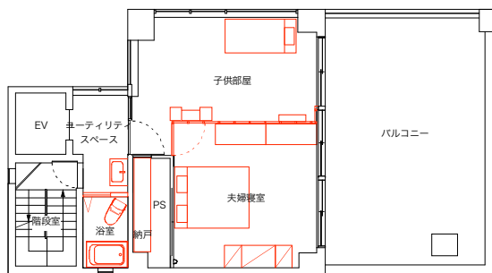
平面図 1/200
